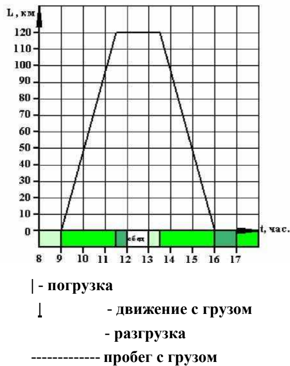
Рис. 3. График движения автомобилей на маршруте
