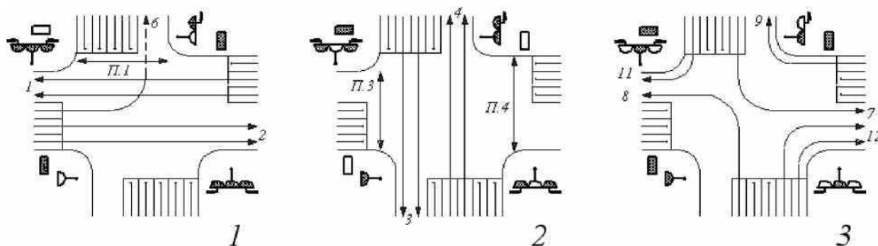
Рис. 1. Организация движения на перекрестке: пофазный принцип управления движением
