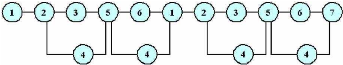
Рис. 2. Технологическая схема перевозки грузов: 1 - движение автомобиля к пункту погрузки; 2 - ожидание погрузки, маневрирование; 3 - погрузка; 4 - оформление документов на груз; 5 - движение автомобиля к пункту разгрузки; 6 - разгрузка; 7 - движение автомобиля на стоянку
