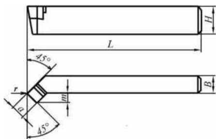
Рис. 2 - Резец токарный проходной, отогнутый с пластинами из твердого сплава (ГОСТ18877-73)
